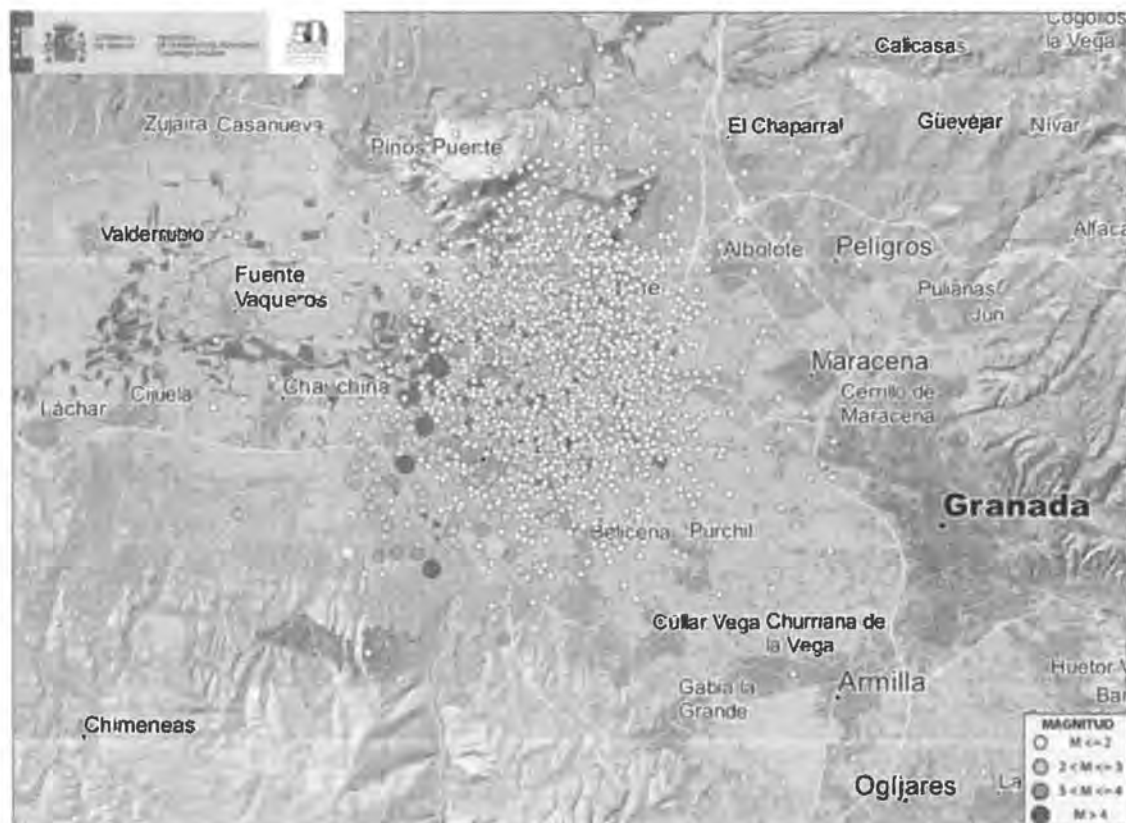
Figura 1. Mapa de sismicidad de la zona epicentral desde el 1 de diciembre de 2020. Fuente: IGN.
