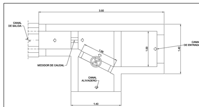
Figura 1.- Planta arqueta de entrada.
