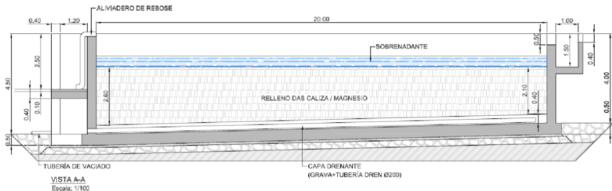
Figura 2.- Tanque reactivo.
